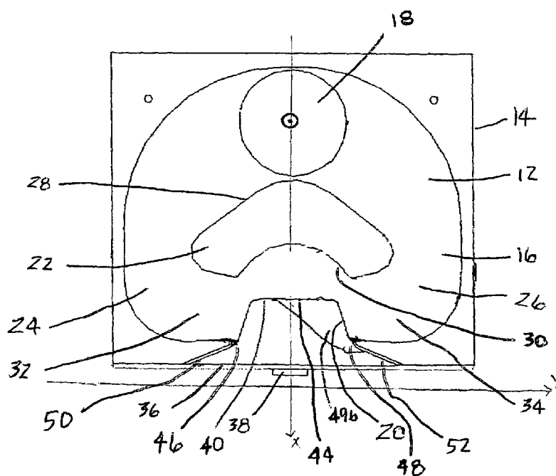
FIG. 11 Section 1-1
