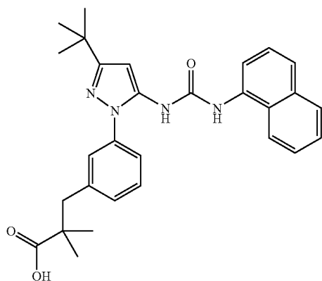
Example 224
