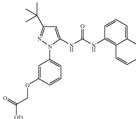
Example 186
