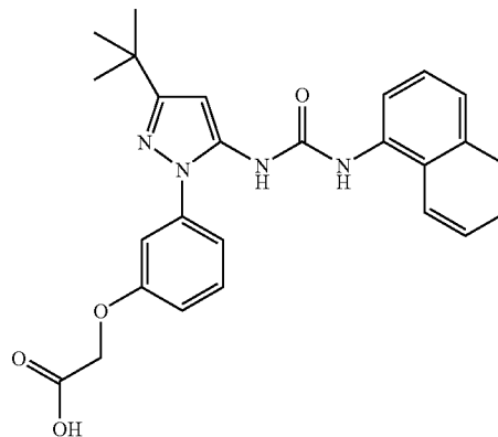
Example 187
