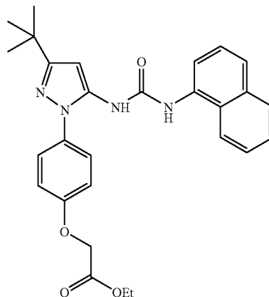
Example 190
