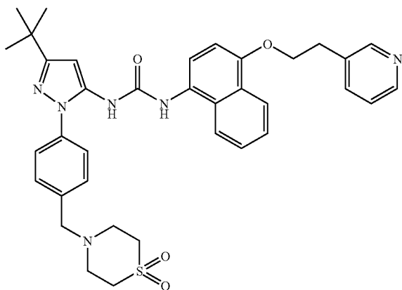
Example 119
