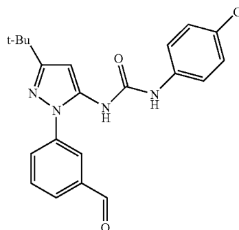
Example 243
