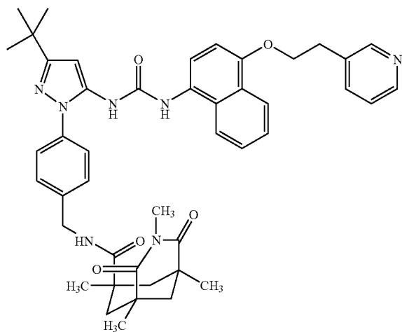
Example 113
