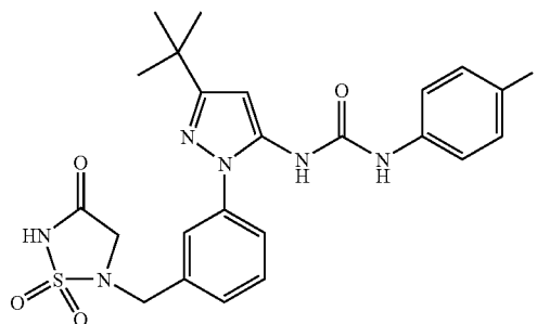
Example 162
