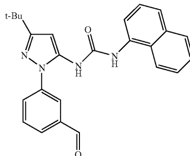
Example 241
