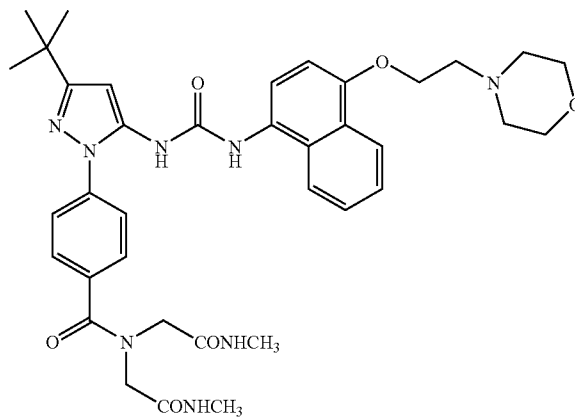
Example 127
