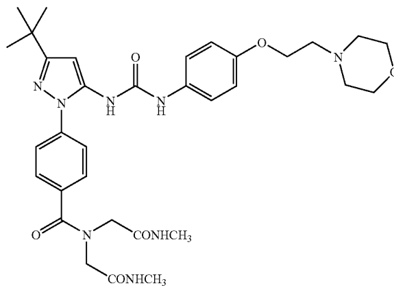
Example 128
