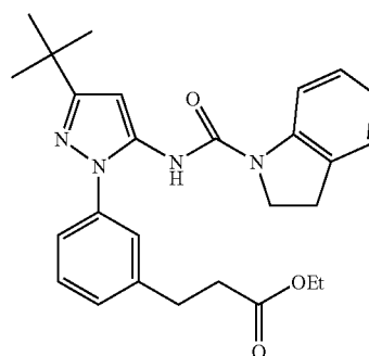
Example 176
