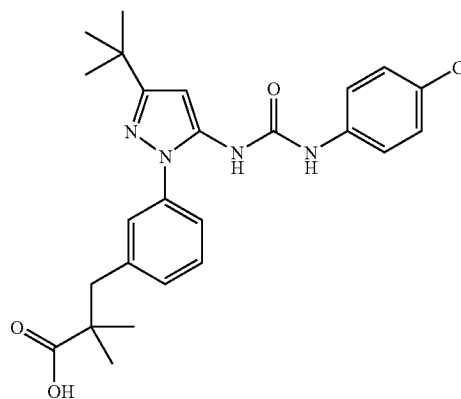
Example 226
