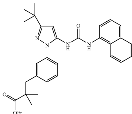
Example 223
