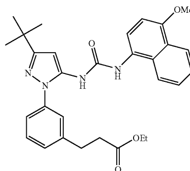
Example 174
