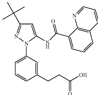
Example 222
