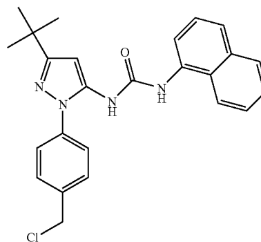
Example TT
