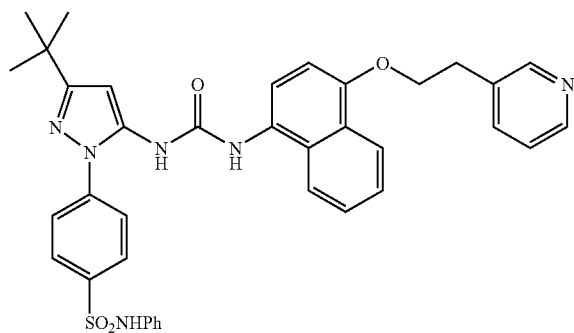
Example 137
