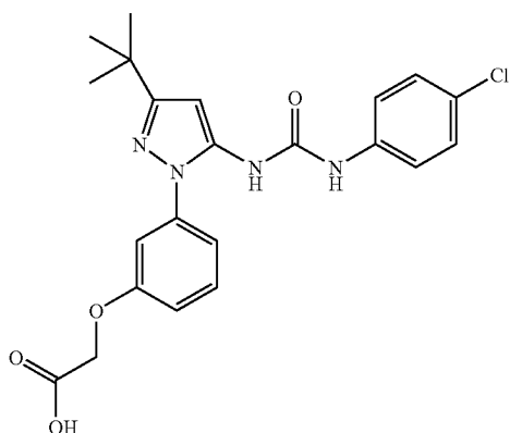
Example 189
