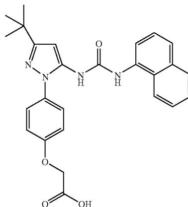
Example 191
