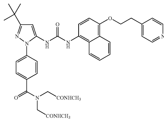
Example 129
