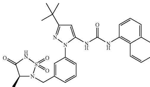
Example 161
