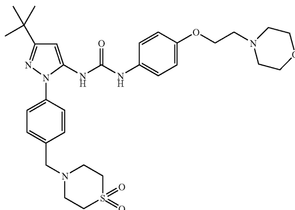
Example 116
