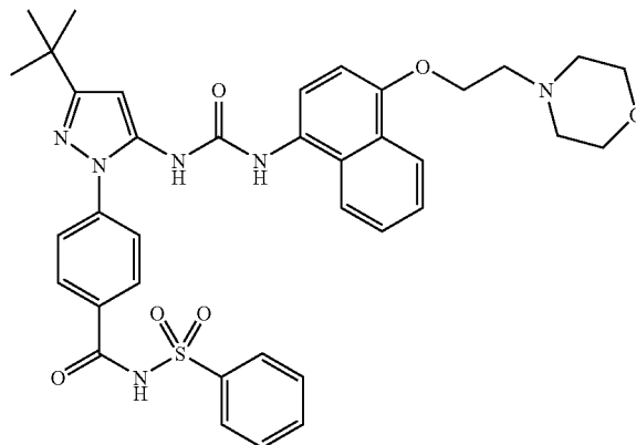
Example 121
