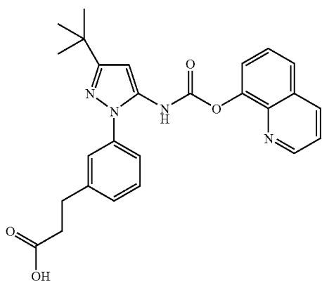
Example 173
