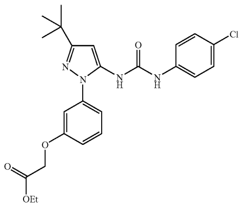
Example 188
