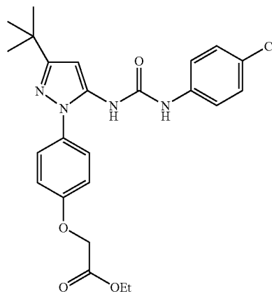
Example 192
