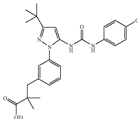
Example 225
