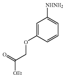
Example OO
