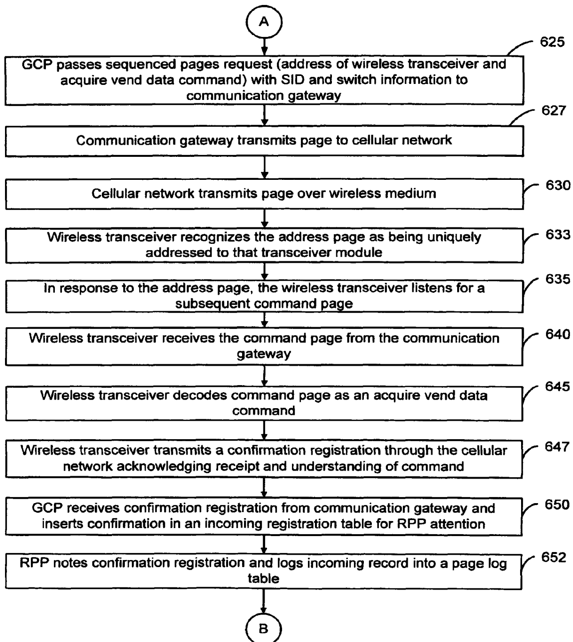
Fig. 6B
