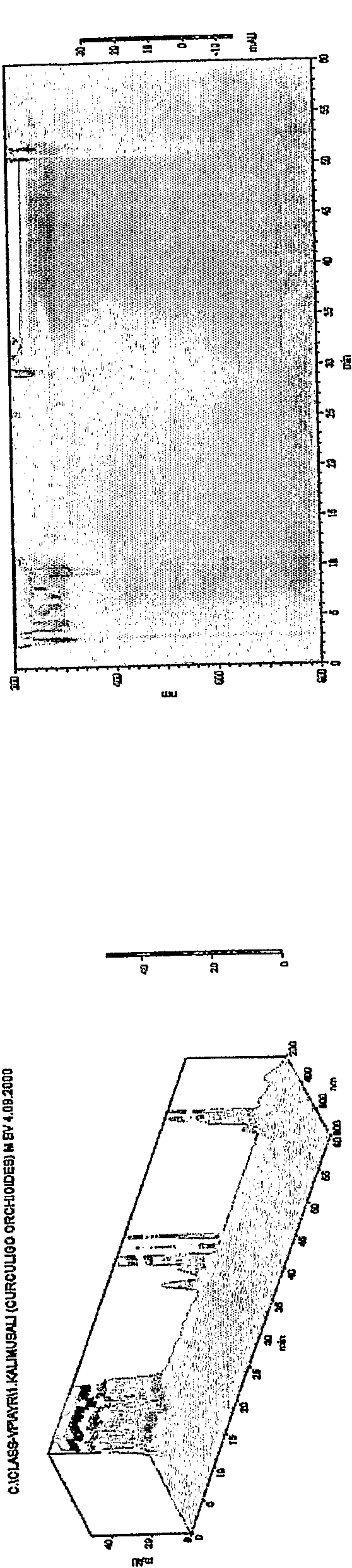
FINGER PRINTS OF CURCULIGO ORCHIOIDIS (KALIMUSALI)
