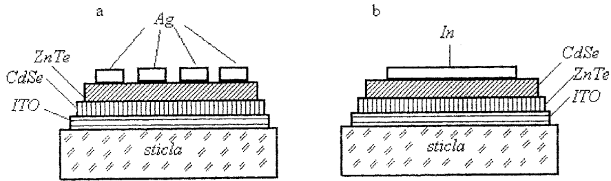
Structura – test a heterostructurii cu straturi subțiri
