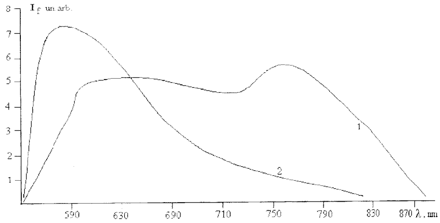
Distribuția spectrală a heterostructurilor lor ZnTe-CdSe : 1 – HS de tip I 2 – HS de tip II
