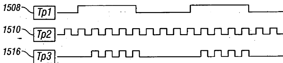
FIG. 16
