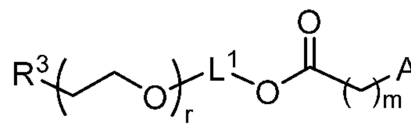
(VII-b-2),
