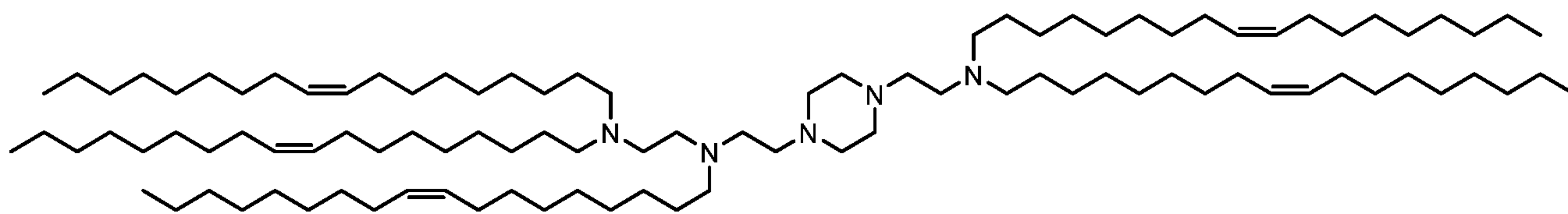
(Compound 342).
