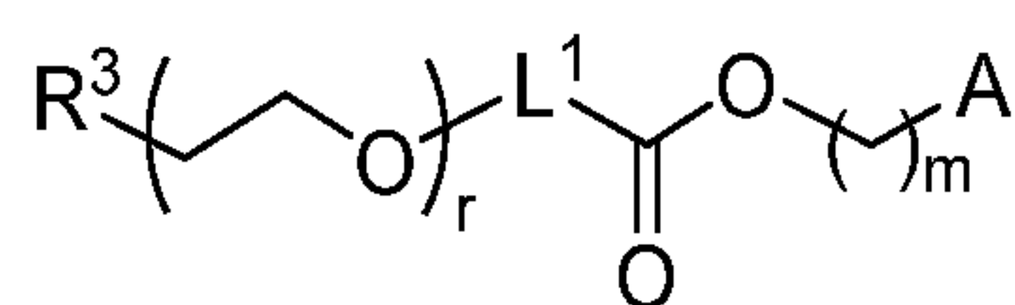
(VII-b-1)
