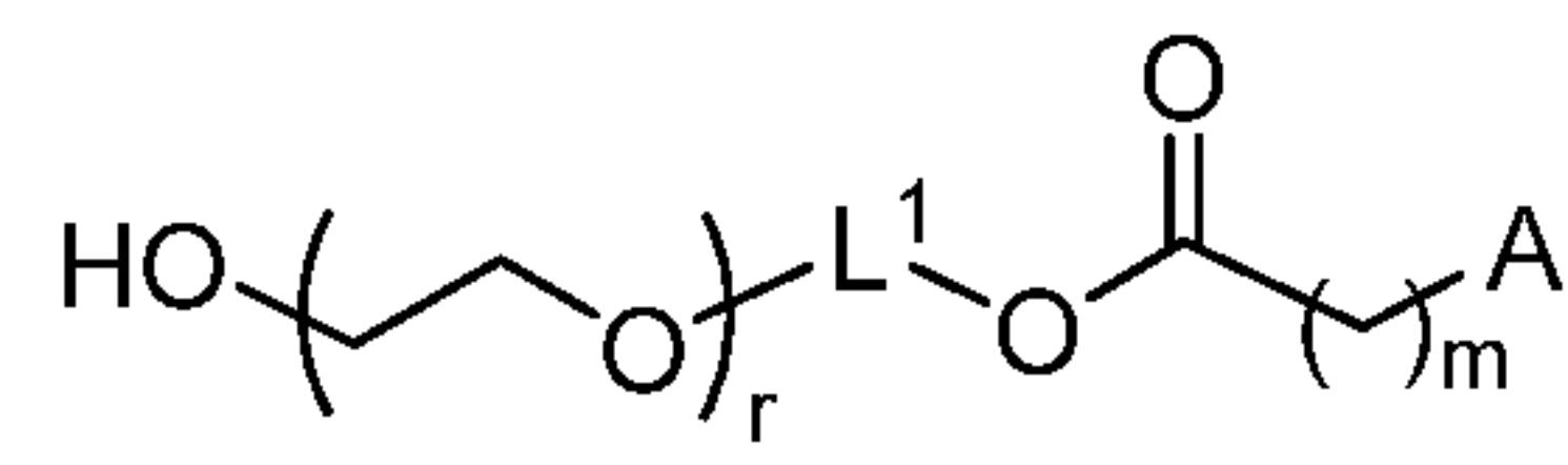
(VII-b-2-OH),
