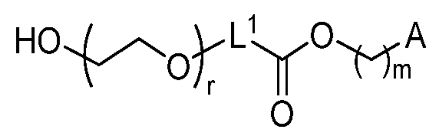
(VII-b-1-OH)
