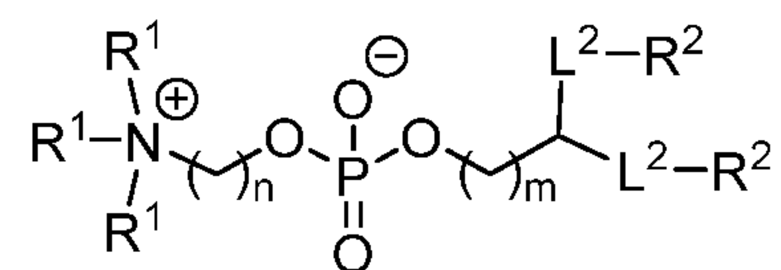
(IX-a),
