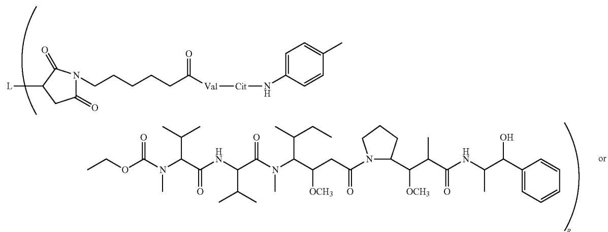
L-MC-vc-PAB-MMAE
