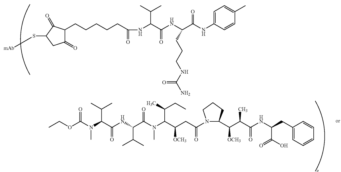
L-MC-vc-PAB-MMAF
