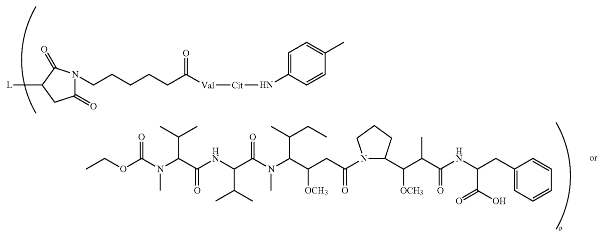
L-MC-vc-PAB-MMAF
