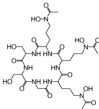
desferrirhodin
