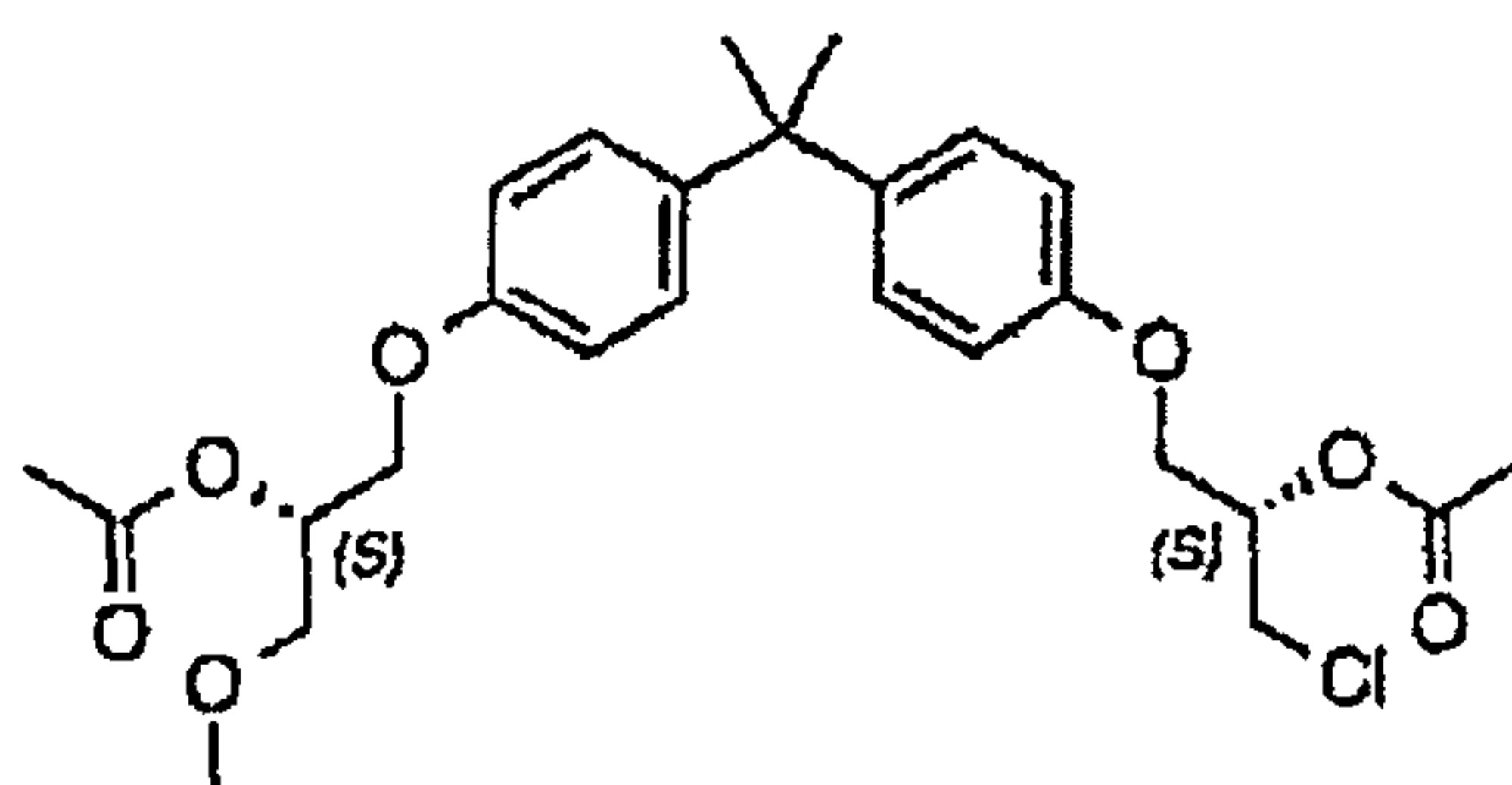
(S)-1-(4-(2-(4-((S)-2-acetoxy-3-chloropropoxy)phenyl)propan-2-yl)phenoxy)-3-methoxypropan-2-yl acetate (Example 21)
