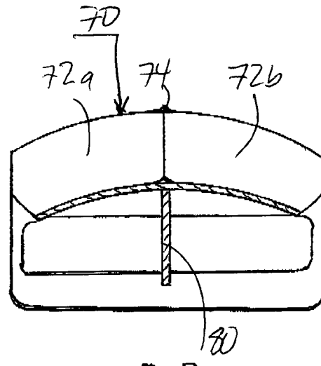
B-B FIG. 22
