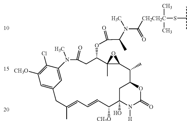
DM4
