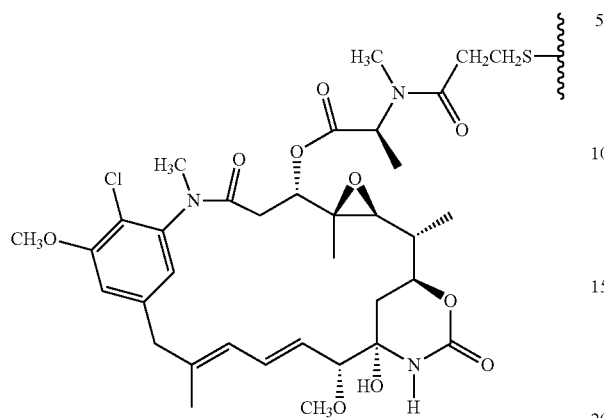
DM3
