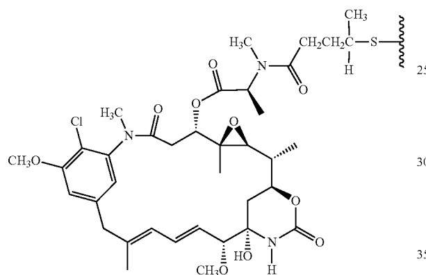
DM3
