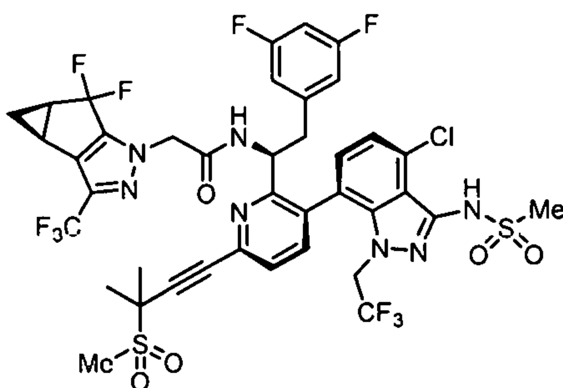
Isomer B.
