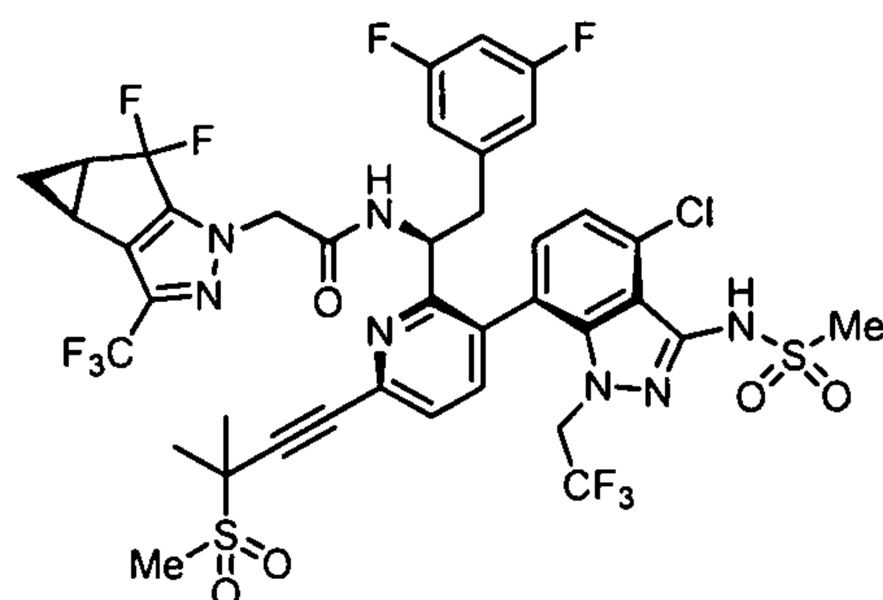
Isomer A.
