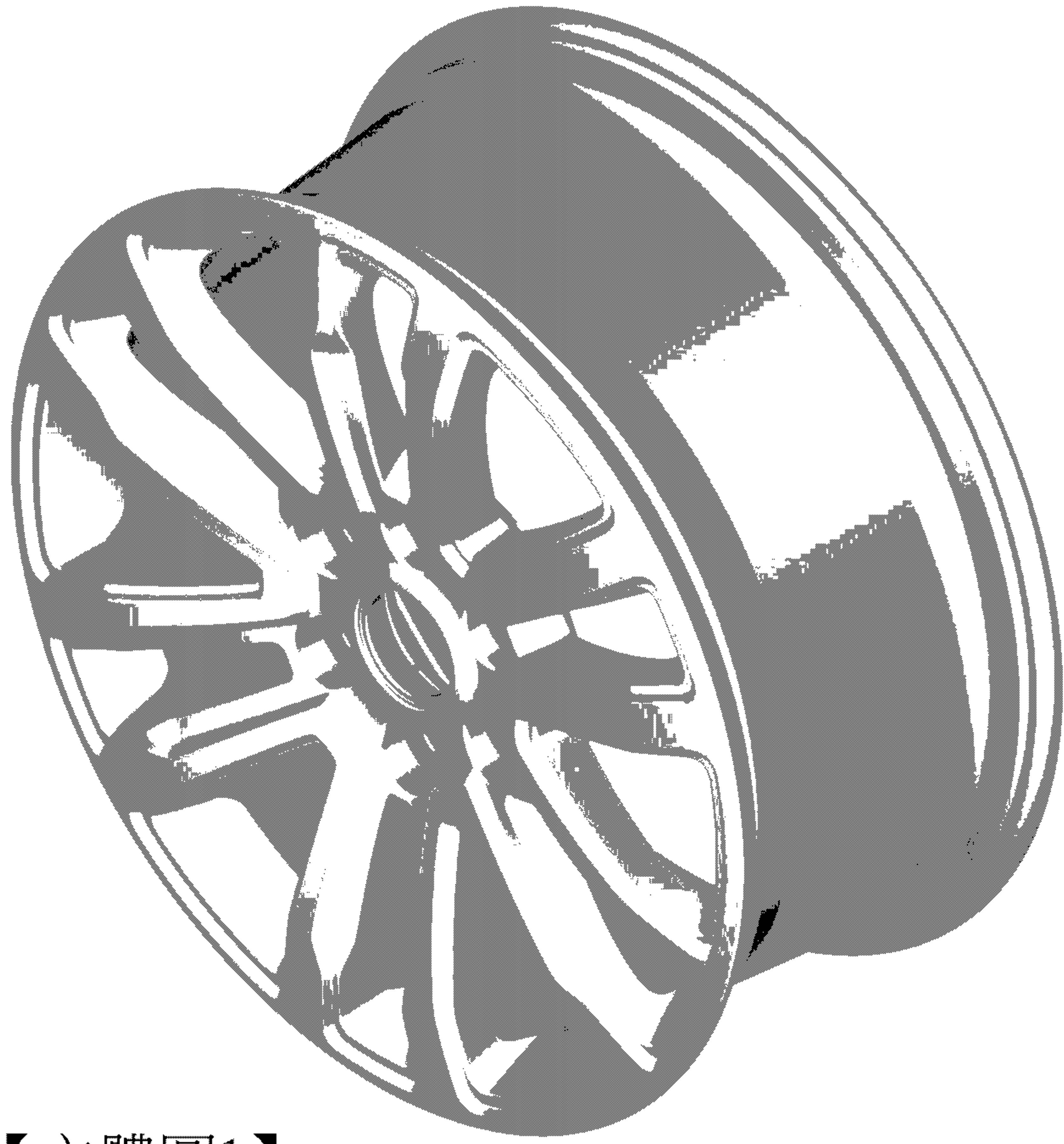
【立體圖1】
