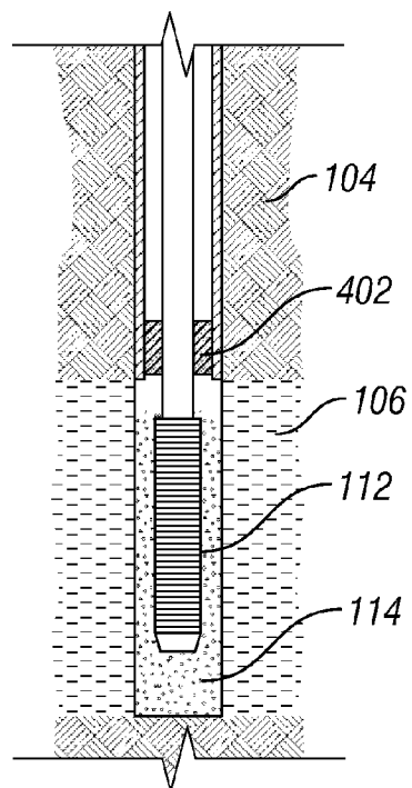
FIG. 4C
