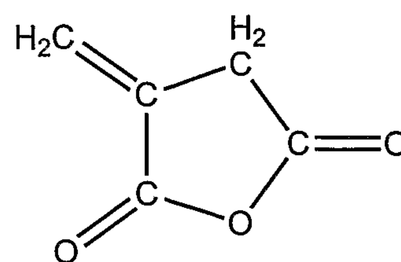
Itaconic Anhydride
