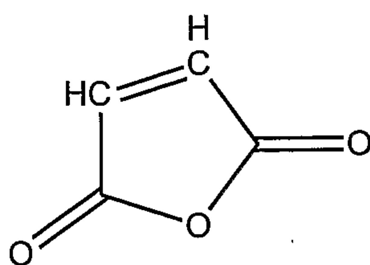
Maleic Anhydride
