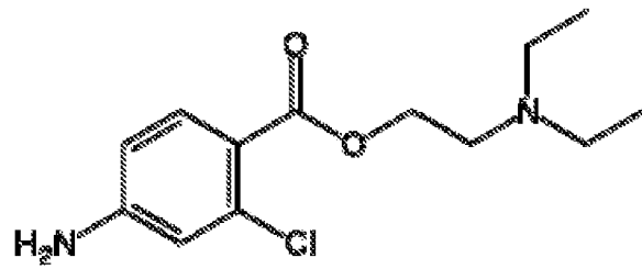
CHLOROPROCAINE
