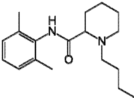
BUPIVACAINE
