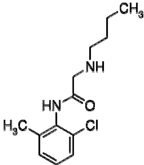
BUTANILCAINE
