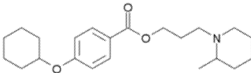
CYCLOMETHYCAINE
