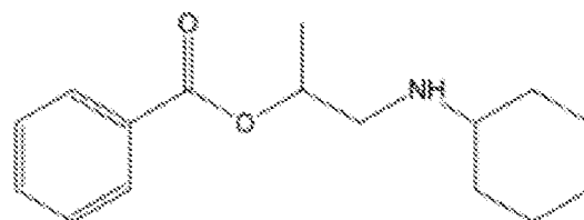
HEXYLCAINE
