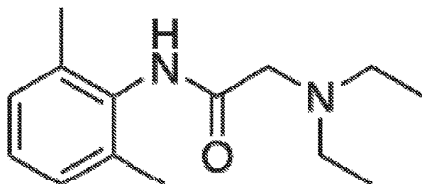
LIDOCAINE
