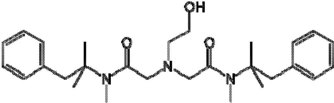
OXETACAINE
