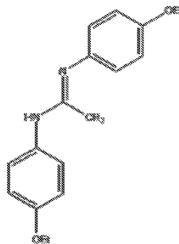
PHENACAINE
