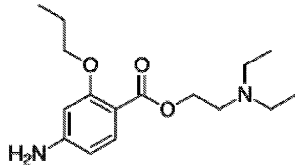
PROPOXYCAINE
