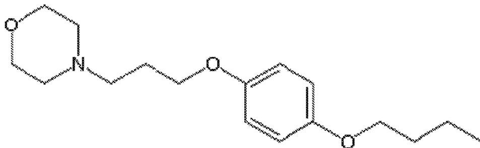
PRAMOCAINE
