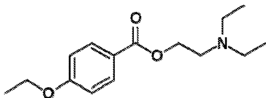
PARAETHOXYCAINE
