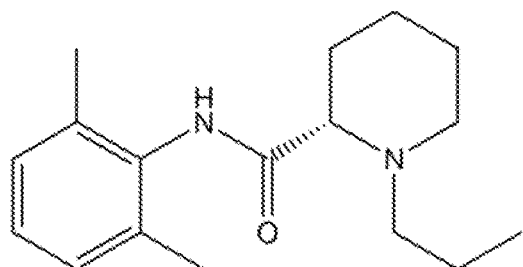
ROPIVACAINE
