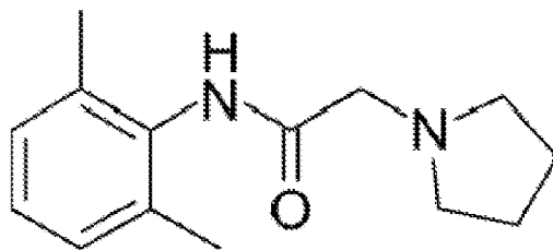
PYRROCAINE
