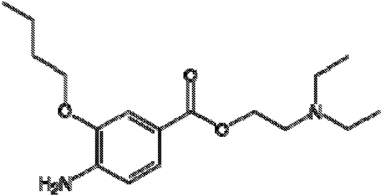
OXYBUPROCAINE
