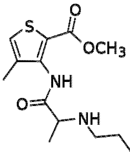
ARTICAINE
