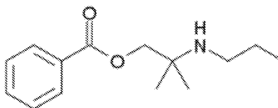
MEPRYLCAINE
