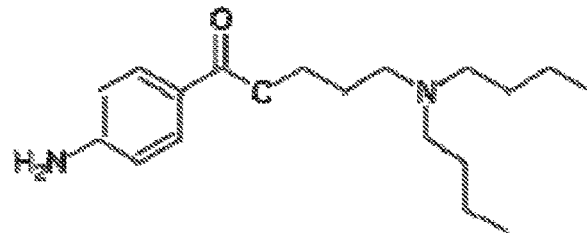
BUTACAINE
