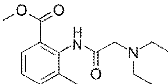
TOLYCAINE
