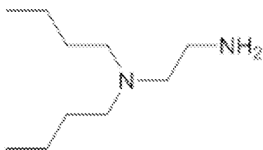
N 1 ,N 1 -dibutylethane-1,2-diamine
