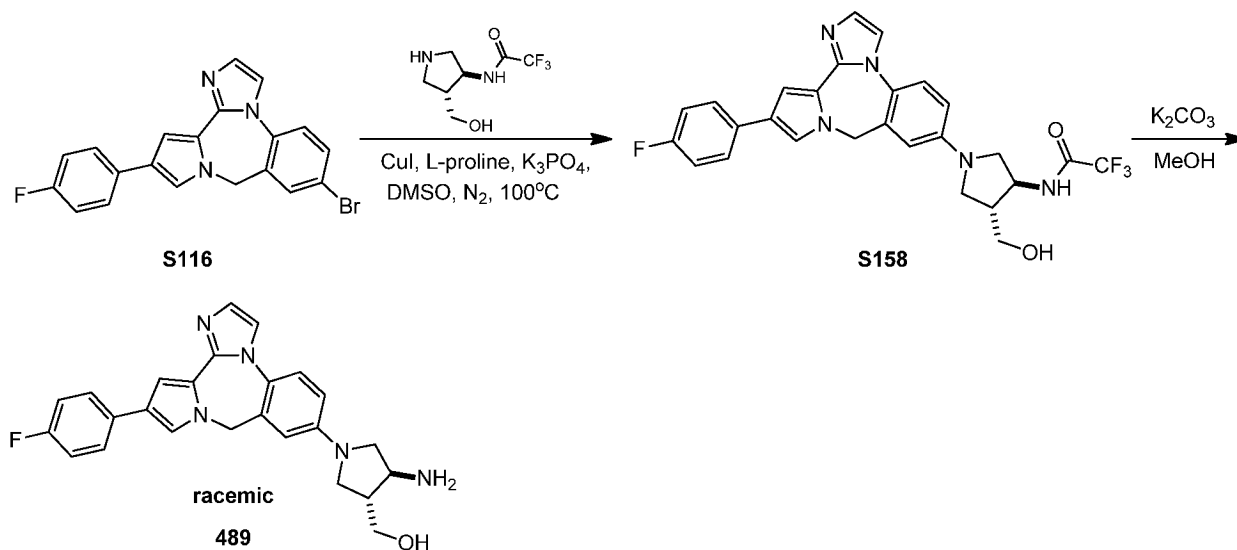
Scheme 43 :
