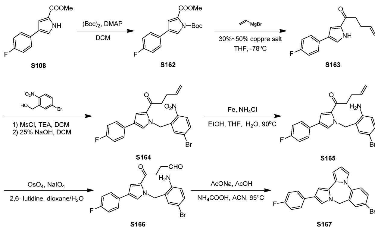
Scheme 47 :
