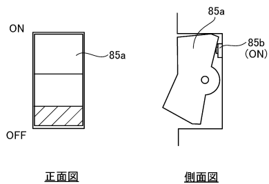
電源スイッチのON状態
