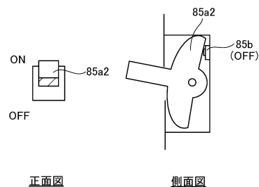
電源スイッチのON状態
