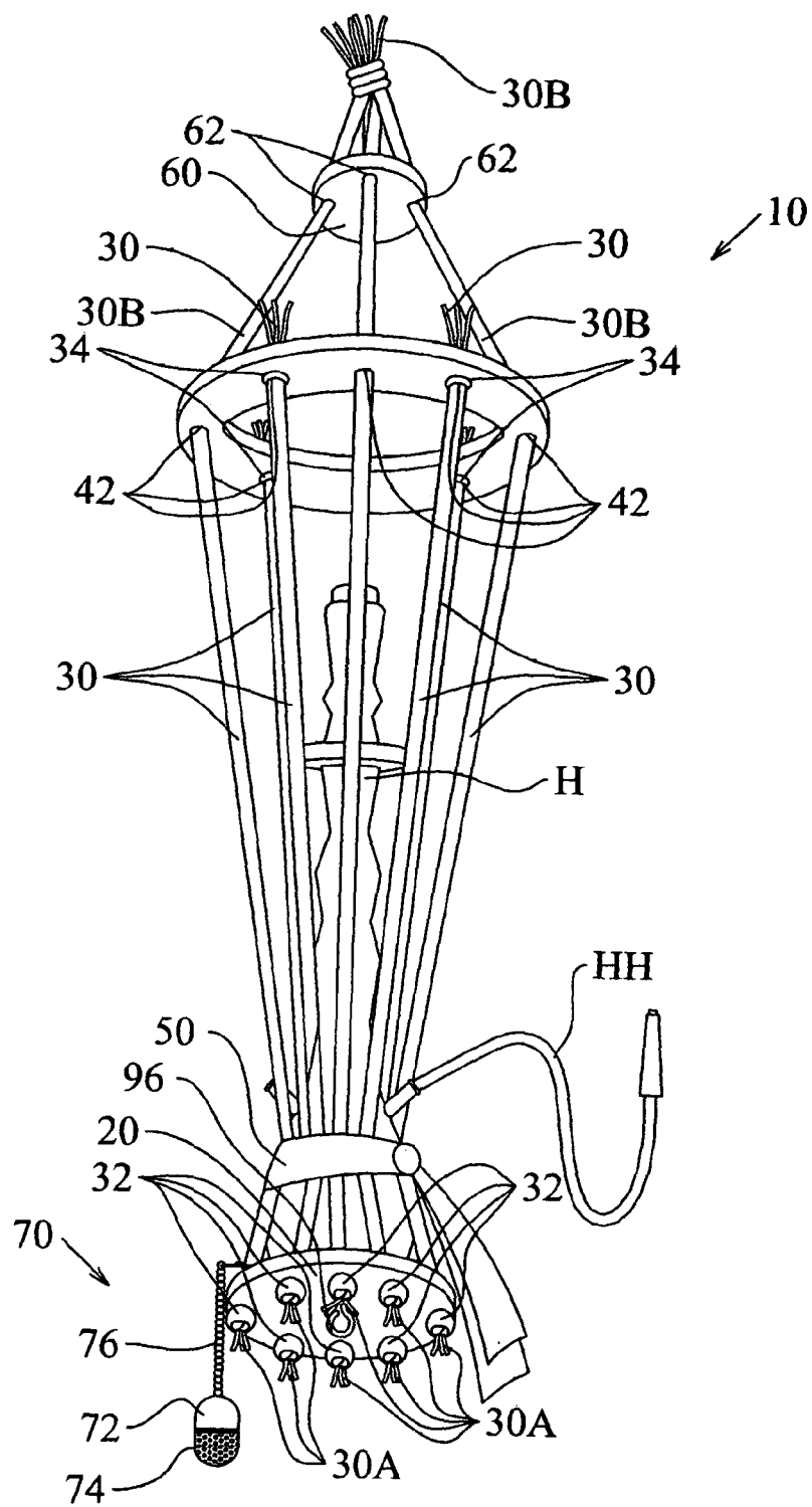
FIG. 3A
