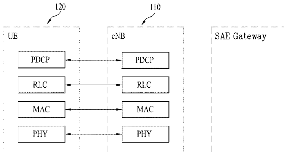
(b) 사용자-평면 프로토콜 스택
