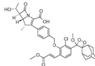
(화학식 VIIa)
