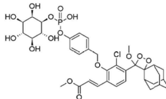
(화학식 IIIa)
