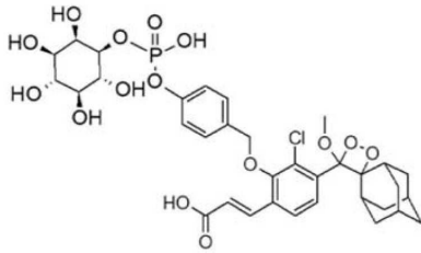
(화학식 IIIb)
