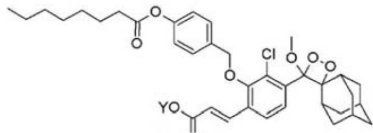
(화학식 II)
