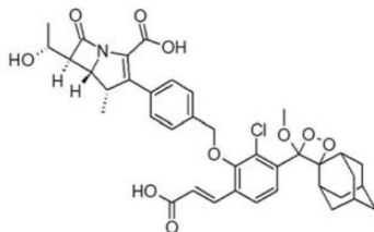
(화학식 VIIb)
