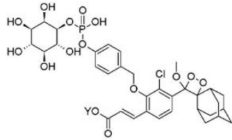
(화학식 III)
