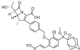
(화학식 VII)
