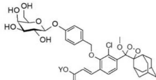
(화학식 V)
