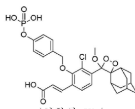
(화학식 IVa)
