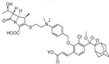
(화학식 VIII)
