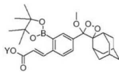
(화학식 VI)
