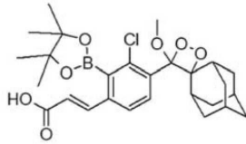
(화학식 VIb)
