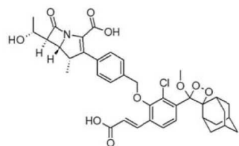
(화학식 VIIb)
