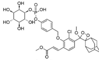
(화학식 IIIa)
