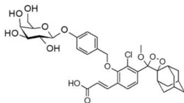
(화학식 Vb)
