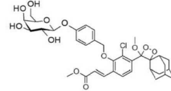
(화학식 Va)
