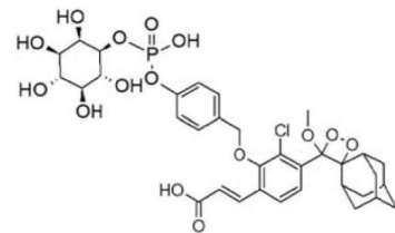
(화학식 IIIb)
