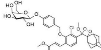
(화학식 Va)
