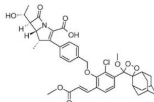
(화학식 VIIa)
