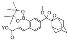
(화학식 VI)
