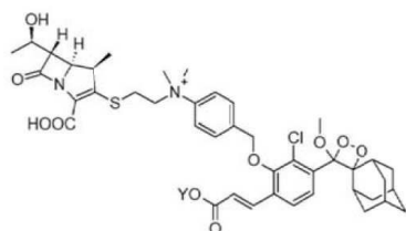
(화학식 VIII)
