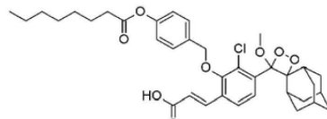
(화학식 IIa)
