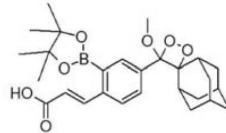
(화학식 VIa)
