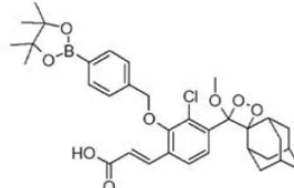
(화학식 VIc)
