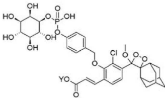
(화학식 III)
