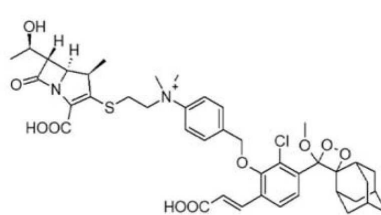
(화학식 VIIIa),
