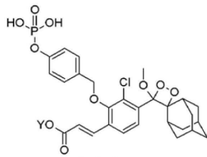
(화학식 IV)
