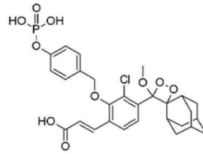
(화학식 IVa)
