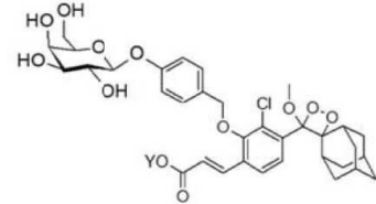
(화학식 V)
