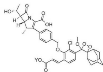
(화학식 VII)
