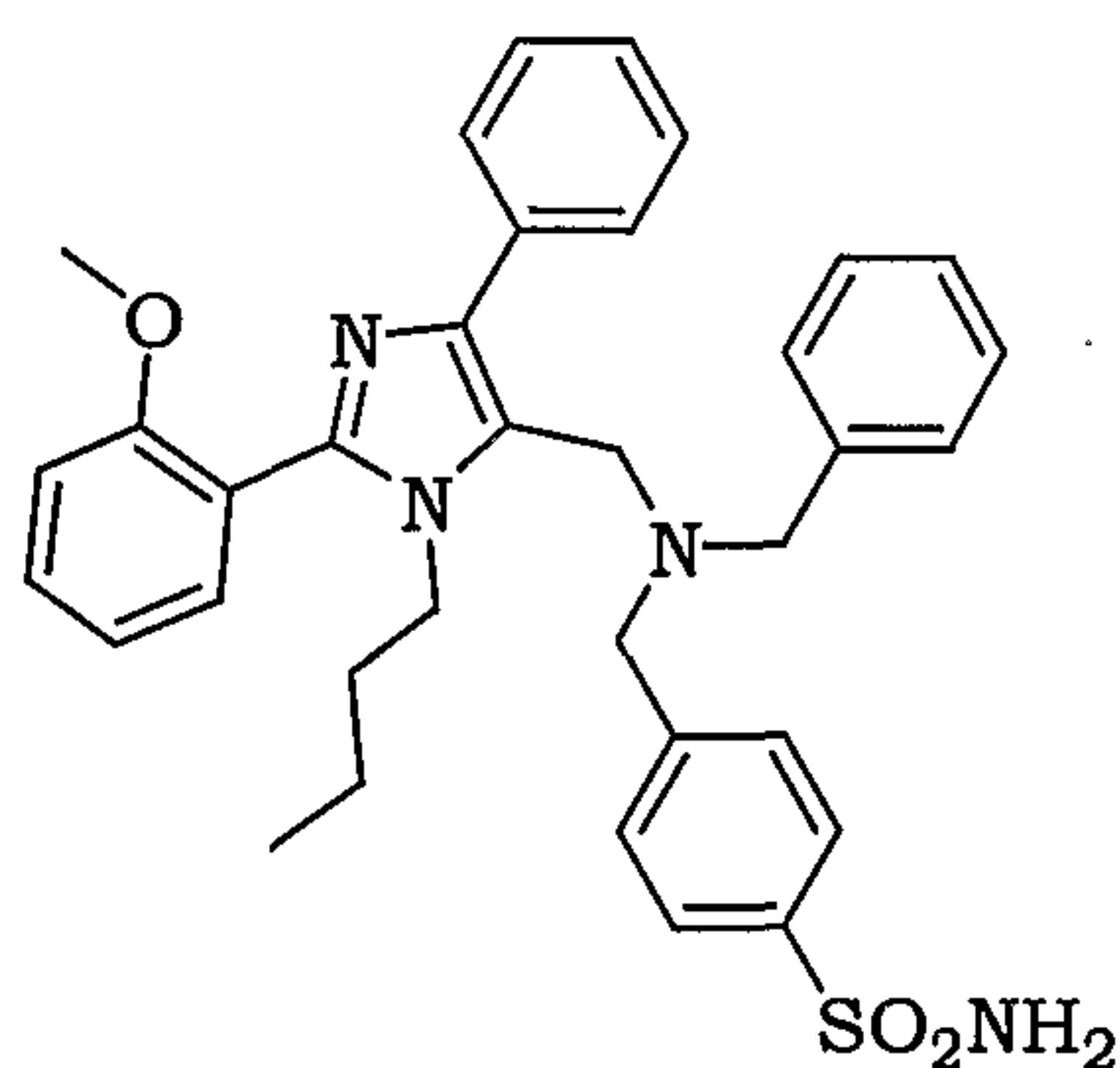
4-({Benzyl-[3-butyl-2-(2-methoxy-phenyl)-5-phenyl-3 H -imidazol-4-ylmethyl]-amino}-methyl)-benzenesulfonamide
