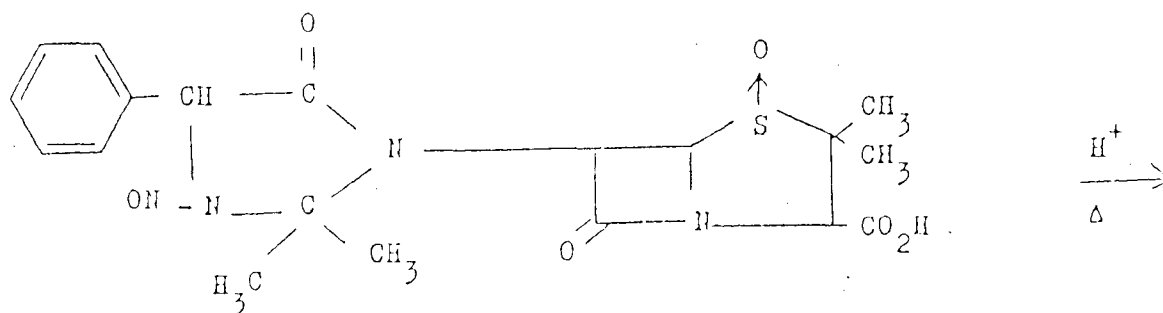
N-nitrosohetasilliini
