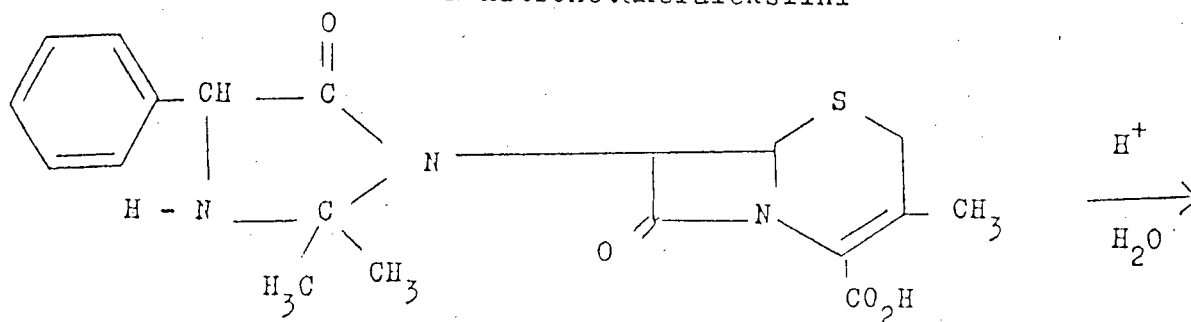
N-nitrohetakefaleksiini
