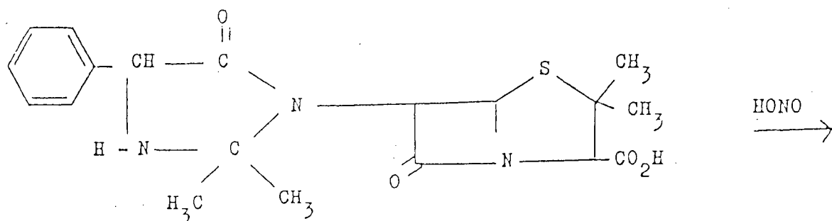
hetasilliini
