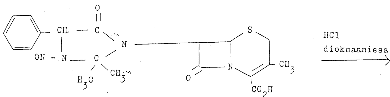
N-nitrohetakefaleksiini
