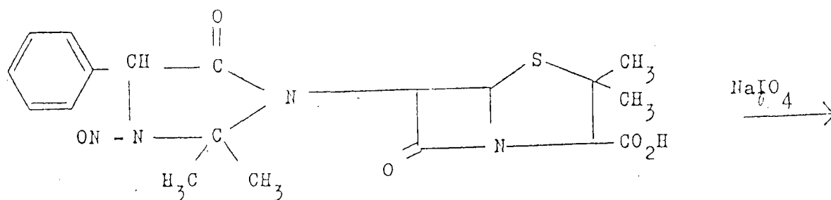
N-nitrosohetasilliini
