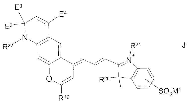
(IIIe)
