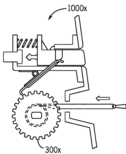
FIG. 8D
