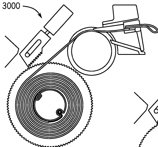
FIG. 16A
