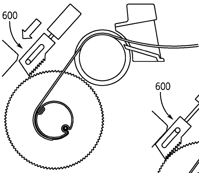
FIG. 16C
