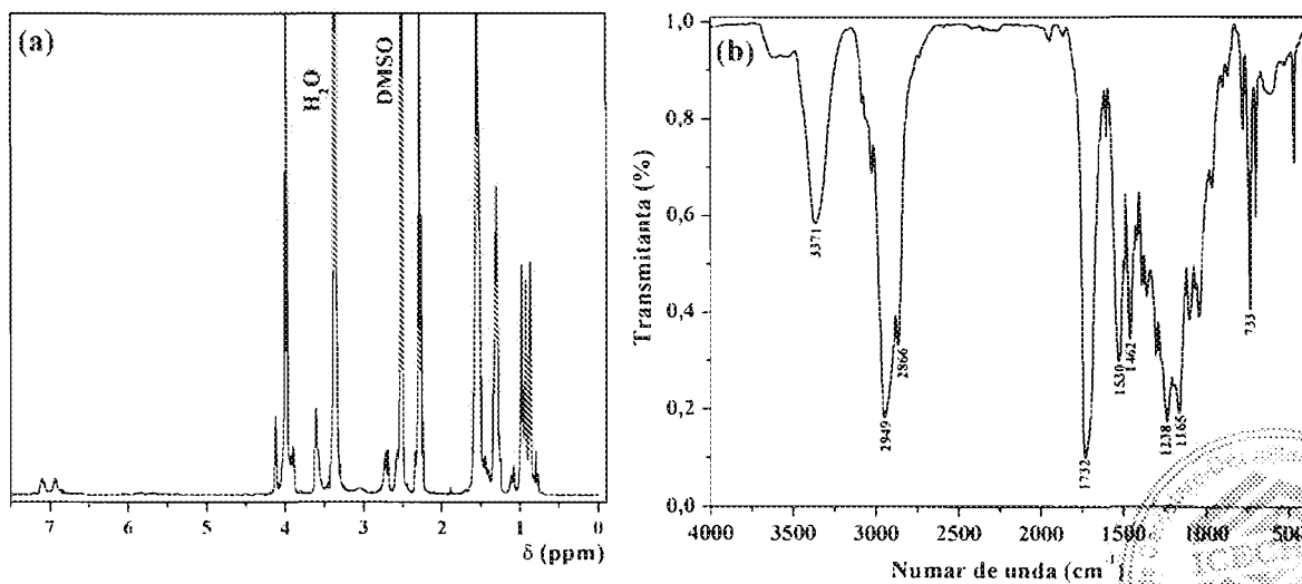
Figura 4. Spectrul ^1\text{H} RMN al PU2 in \text{DMSO-d}_6 (a) si spectrul IR al PU2 (b)
