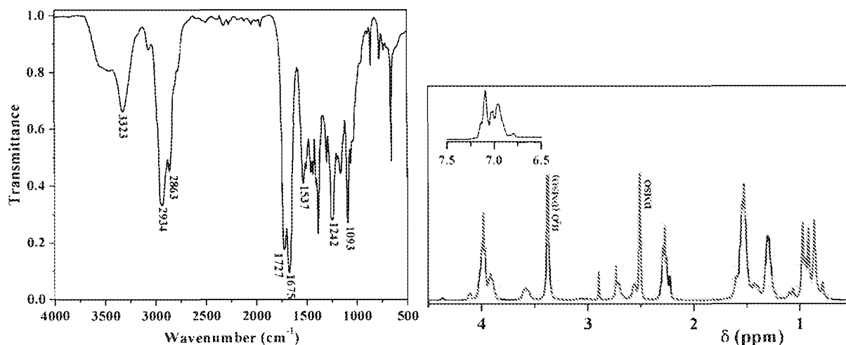
Figura 2. Spectrele IR (stanga) si ^1\text{H} RMN in \text{DMSO-d}_6 (dreapta) ale poliuretanului PU1
