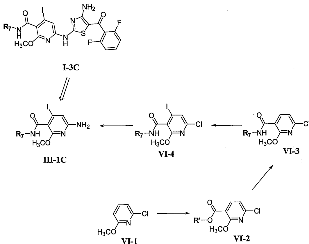
Scheme VI
