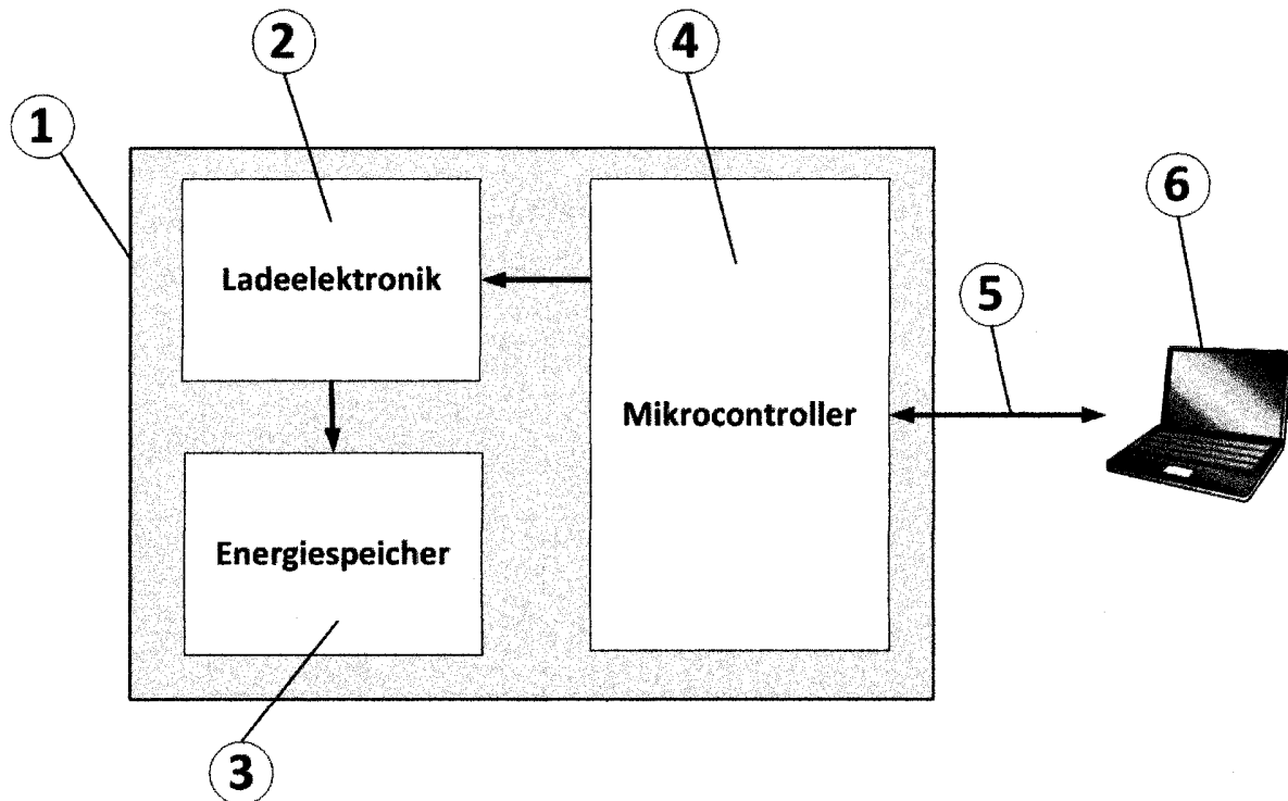
Fig. 1 - Blockschaltbild des bedarfsabhängigen Ladeverfahrens zum optimierten Laden von Energiespeichern
