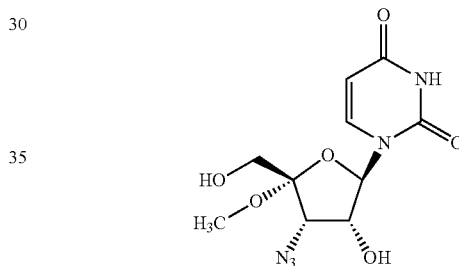
Compound (2e)
