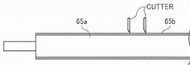
FIG. 18A
