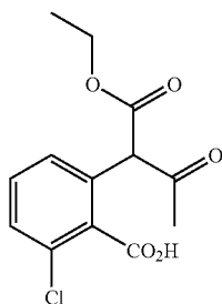
2-Chloro-6-(1-ethoxycarbonyl-2-oxo-propyl)-benzoic acid
