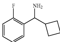
C-Cyclobutyl-C-(2-fluoro-phenyl)-methylamine
