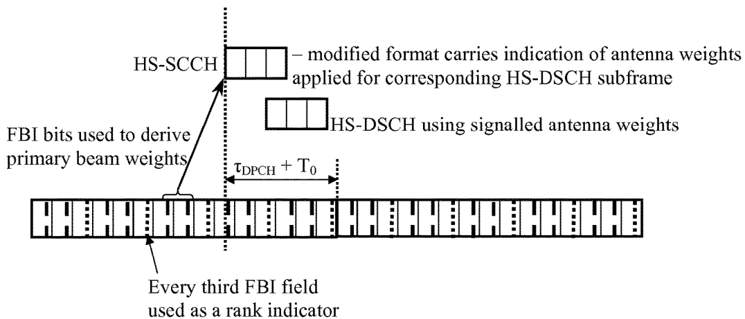
Fig. 2 Use of FBI bits for D-TxAA
