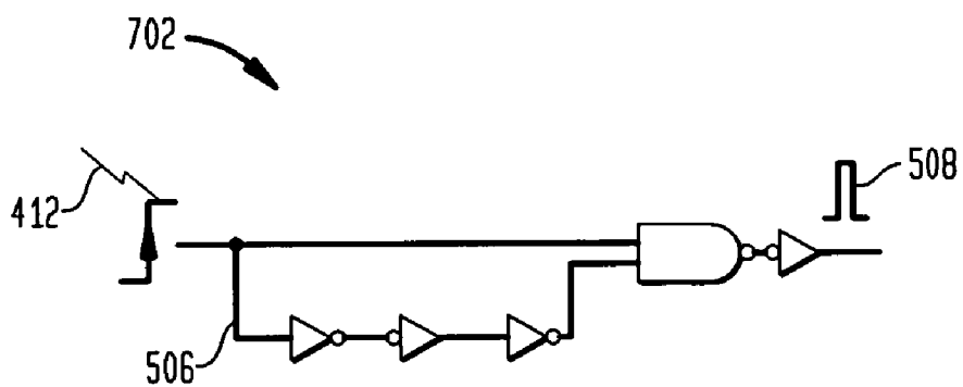
FIG. 7A RISING EDGE PULSE GENERATOR
