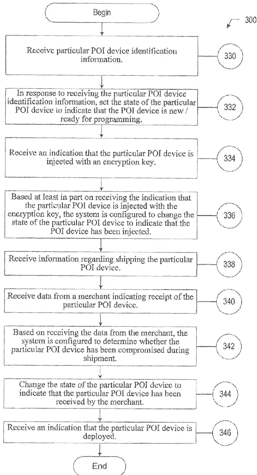
FIG. 3 EXEMPLARY POI HANDLING PROCESS
