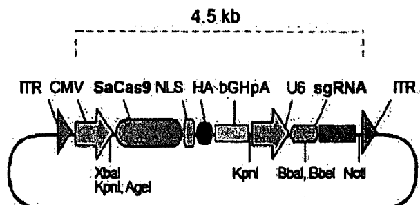
AAV-Sa-Cas9 vector: CMV-SaCas9-NLS-HA-U6-sgRNA
