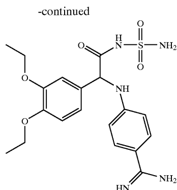
VIIa (Ki) = 0.029 \mu M
