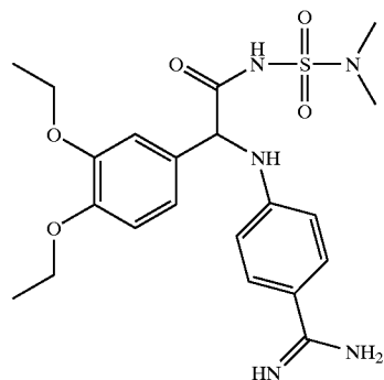
VIIa (Ki) = 0.029 \mu M
