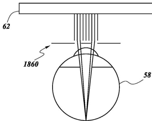
도면18a
