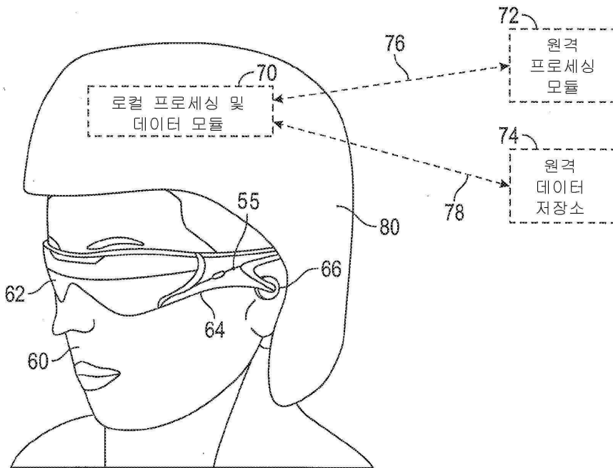
도면3c
