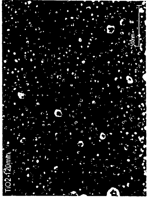
TiO 2 coating 120 min, calcined.
