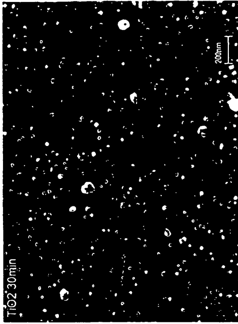
TiO 2 coating 30 min
