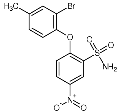
(XIX)
