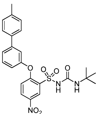
(XLI) Mw - 483.54
