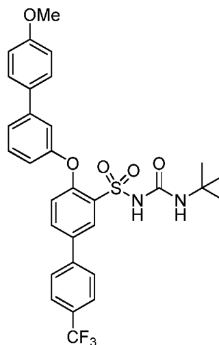
(XLIX) Mw - 598.63
