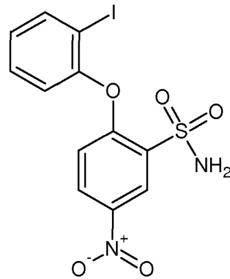
(XVII)
