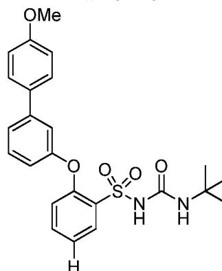
(LIII)
