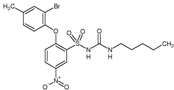
(III)
