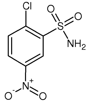
(XV)
