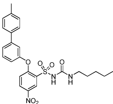
(IX) Mw - 497.56
