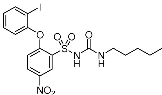
(XXIV) Mw - 533.34
