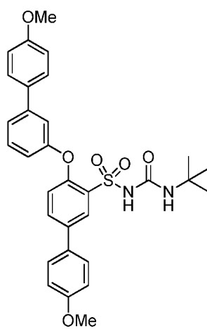
(LVI)
