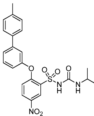
(XXXIX) Mw - 469.51
