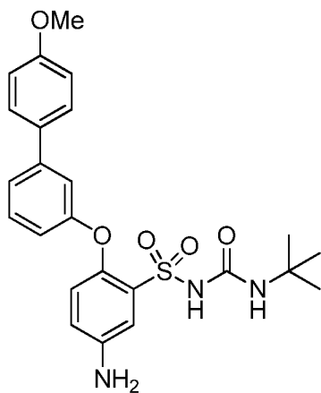
(LII)
