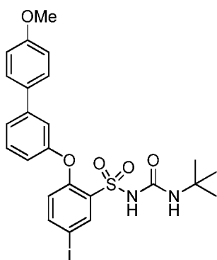
(LIV)
