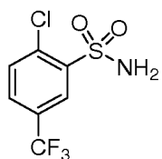
(XVI) Mw - 259.63
