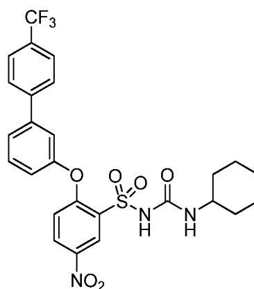
(XXV) Mw - 563.55
