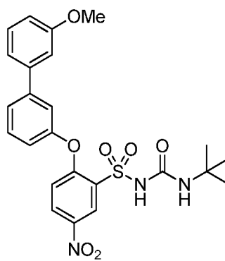
(XLIV)
