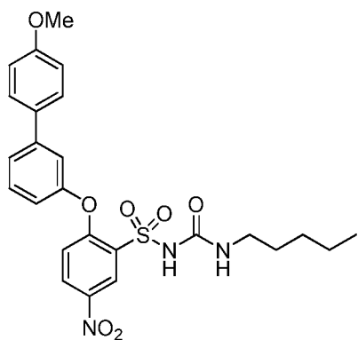
(XLIII)
