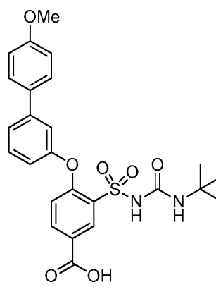
(LV)
