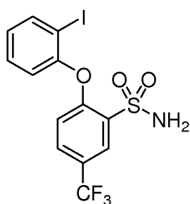
(XVIII) Mw - 443.18
