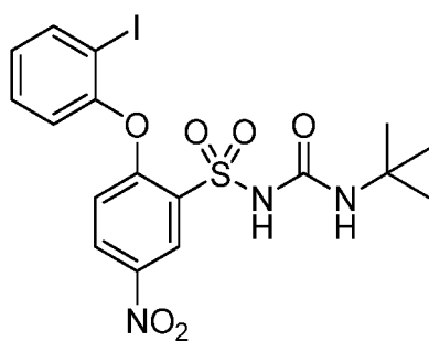
(VIII) Mw - 519.31
