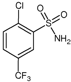
(XVI)
