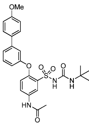
(L) Mw - 511.59
