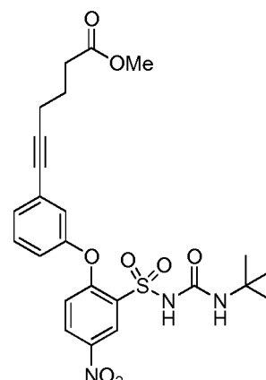
(XXXIII) Mw - 517.55
