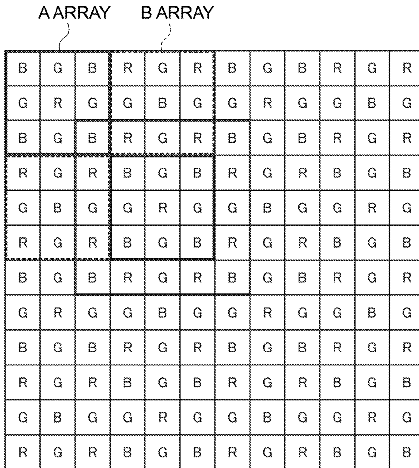
FIG.10A
