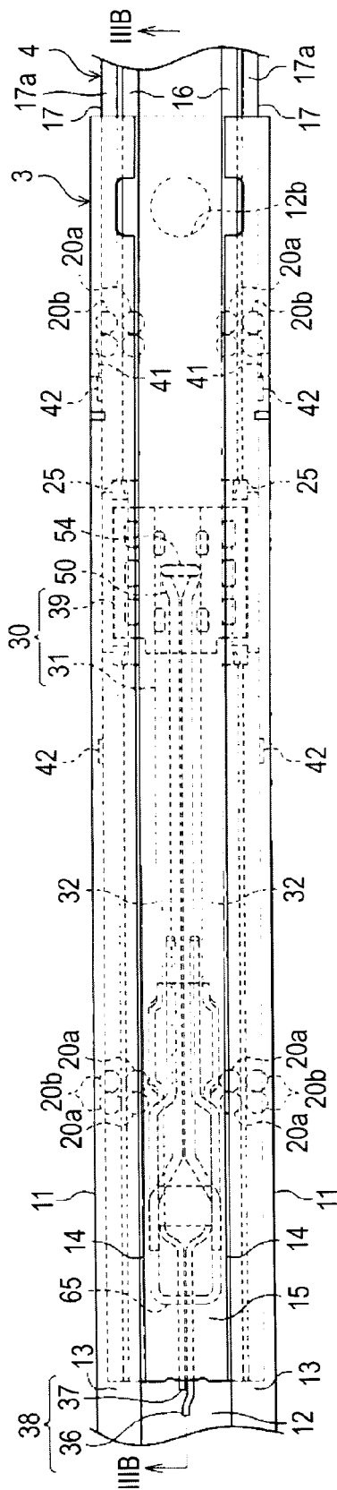
FIG.3A
