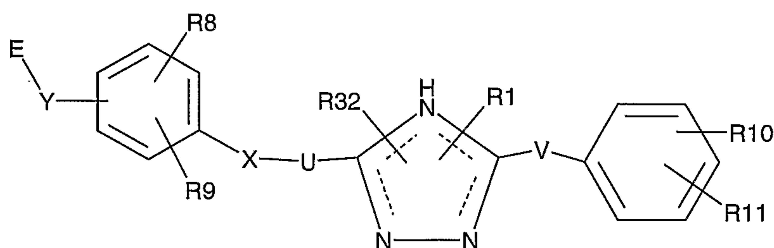
Ia
