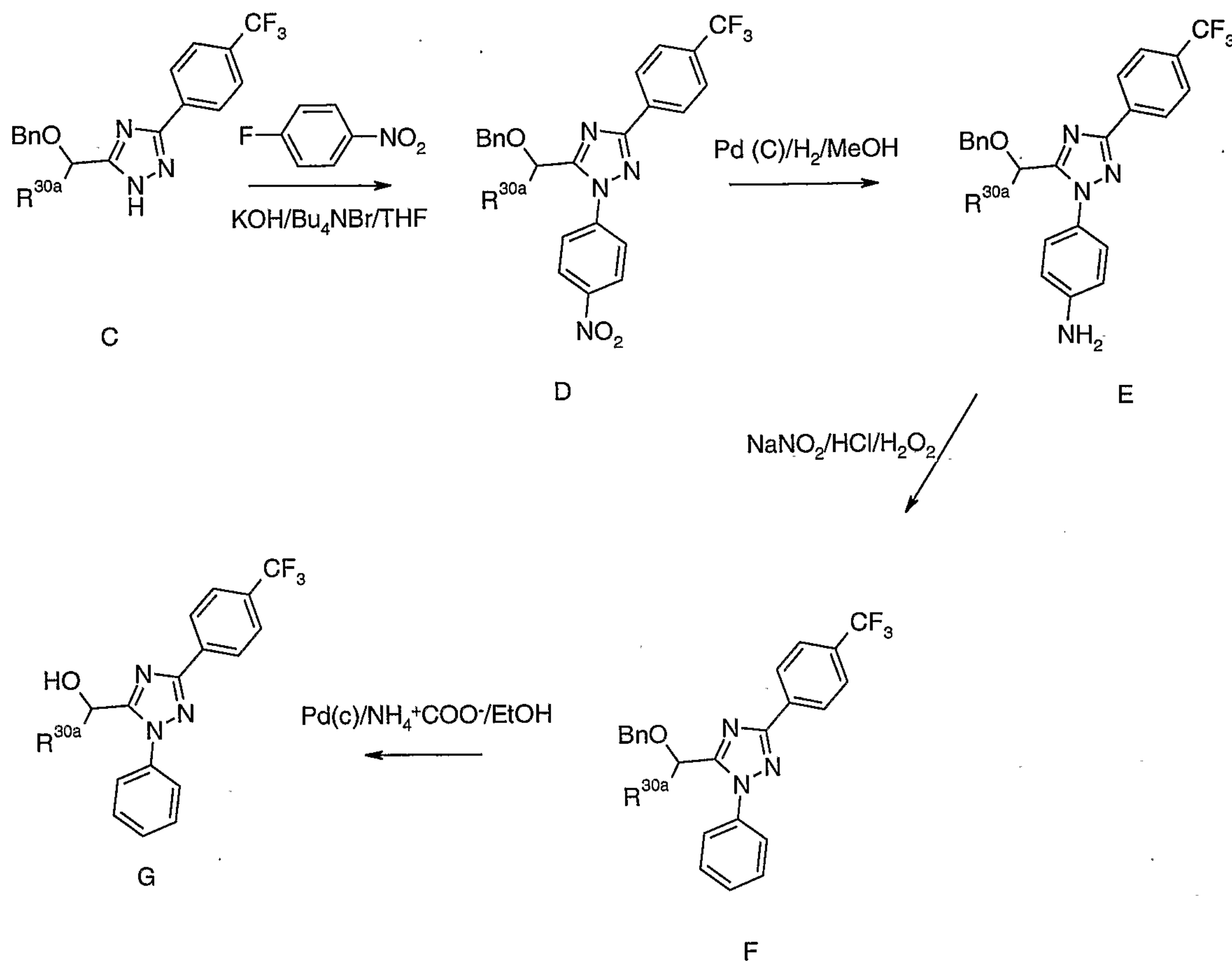
Scheme 2A
