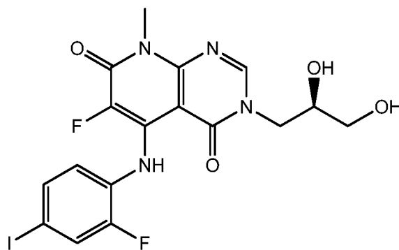
TAK-733
