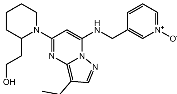
dinaciclib
