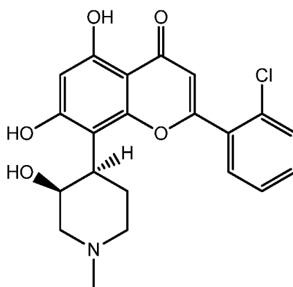
alvocidib
