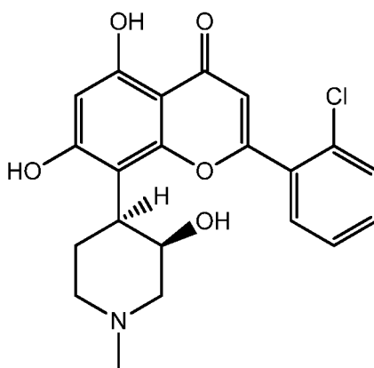
flavopiridol
