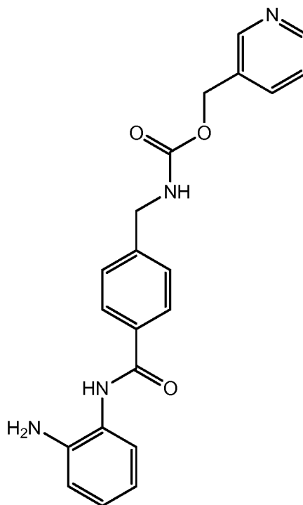
entinostat
