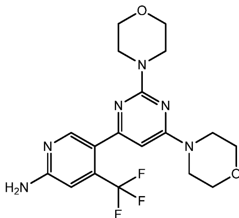
buparlisib
