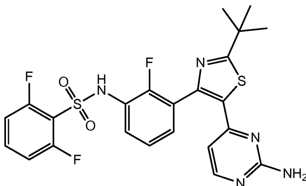
dabrafenib
