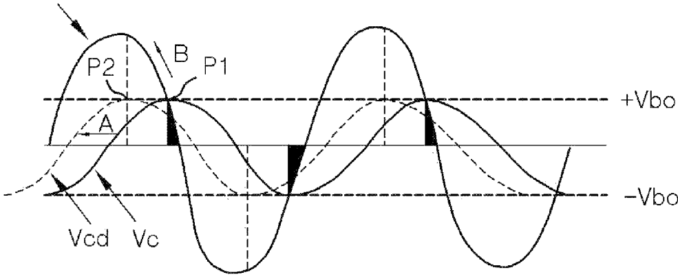
FIG. 5 AC VOLTAGE
