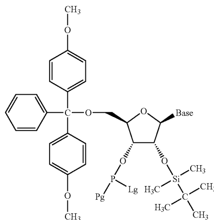
DMT/TBDMS
