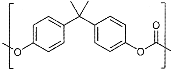
[화학식 4-1]
