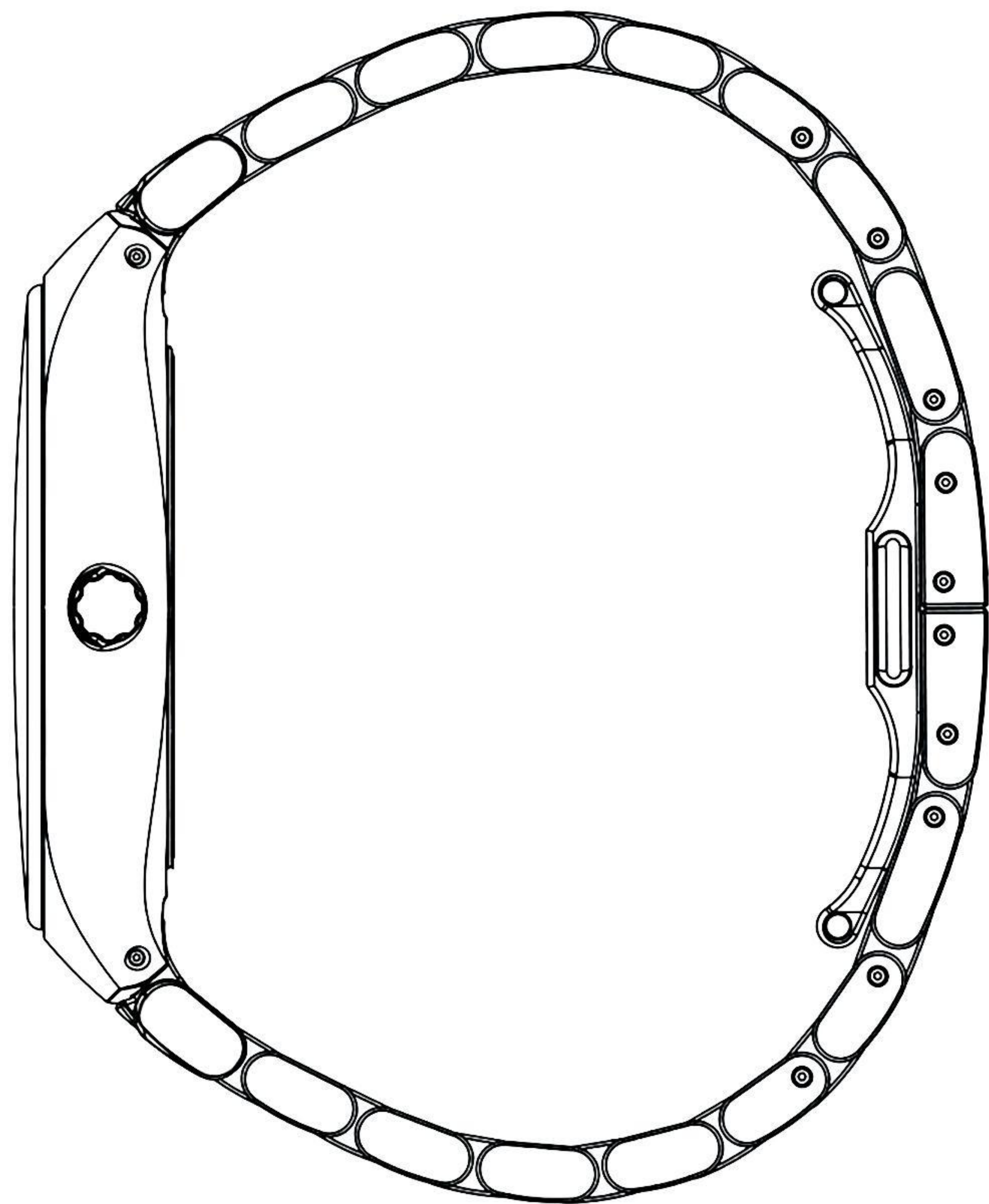
【 右側視圖 】
