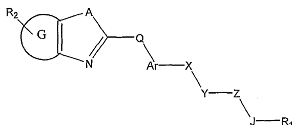
Formula VIIb
